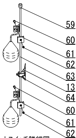
フロートスイッチ詳細図
