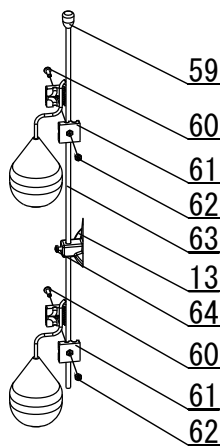
フロートスイッチ詳細図
