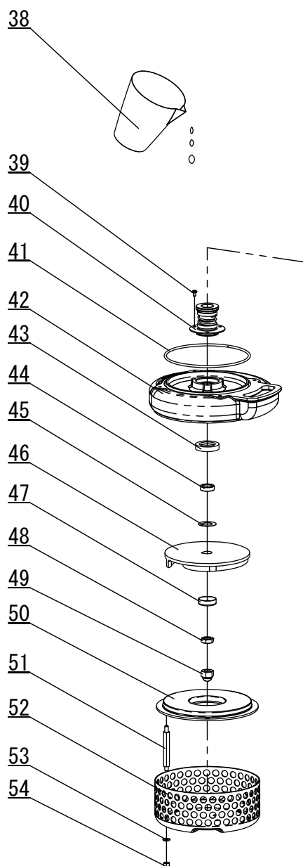
フロートスイッチ詳細図
