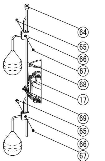
フロートスイッチ詳細図
